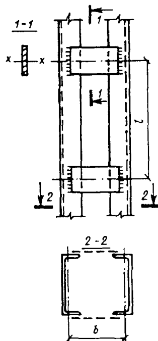
Рис. 3. Составной стержень на планках
