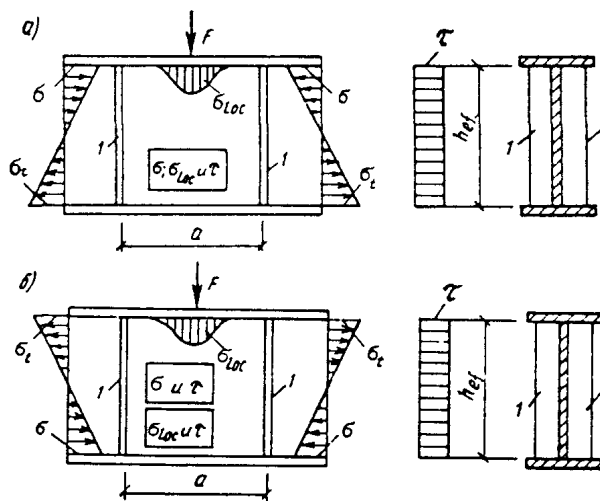
Рис. 12. Схема балки, укрепленной поперечными основными ребрами жесткости (I)
