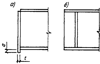
Рис. 15. Схема устройства опорного ребра жесткости
