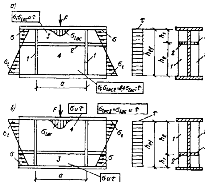
Рис. 13. Схема балки, укрепленной поперечными основными ребрами и продольным ребром жесткости
