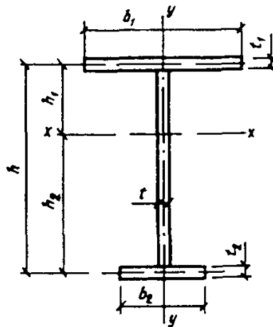
Рис. 28. Схема двутавового сечения с одной осью симметрии при изгибе
