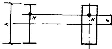
Рис. 16*. Схема внецентренно-сжатых элементов двутаврового и коробчатого сечений
