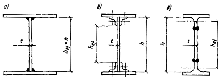
Рис. 10. Расчетная высота стенки составной балки
