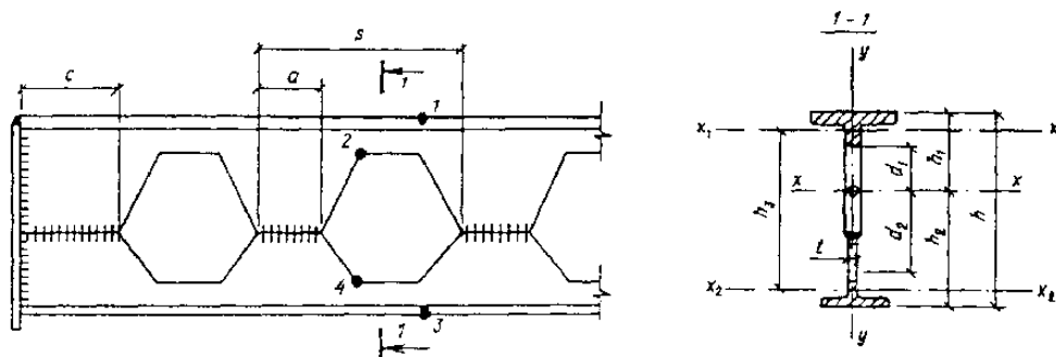
Рис. 23. Схема участка балки с перфорированной стенкой
