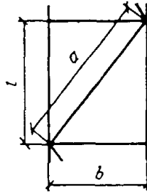
Рис. 2. Схема раскосной решетки
