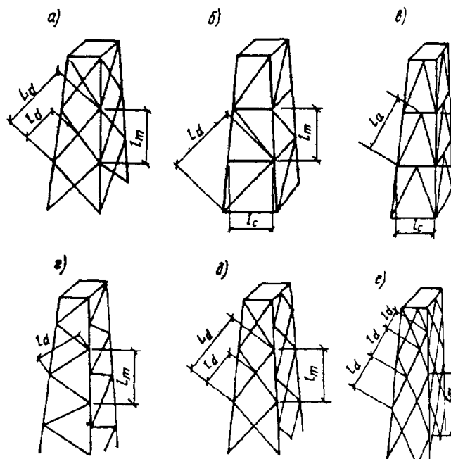
Рис. 9*. Схемы пространственных решетчатых конструкций
