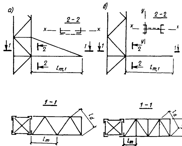
Рис. 21. Схемы траверс
