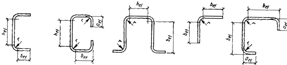
Рис. 11. Схемы поперечных сечений гнутых профилей
