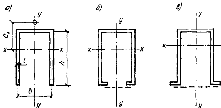
Рис. 1. П-образные сечения элементов
