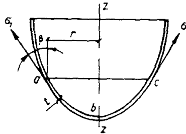
Рис. 17. Схема оболочки вращения
