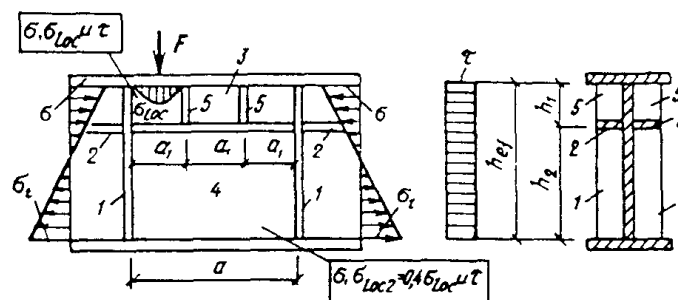
Рис. 14. Схема балки, укрепленной поперечными основными ребрами жесткости (1), продольным ребром жесткости (2), разделяющим отсек стенки на пластинку (3) у сжатого пояса и пластинку (4) у растянутого пояса, а также короткими ребрами жесткости (5)
