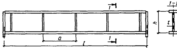
Рис. 22. Схема балки с гибкой стенкой
