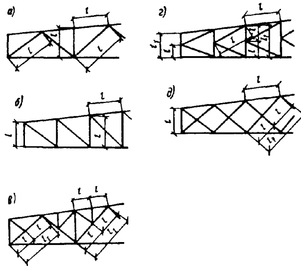
Рис. 7. Схемы решеток ферм для определения расчетных длин элементов
