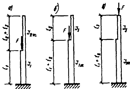
Рис. 26. Схемы одноступенчатых колонн (к табл. 71)
