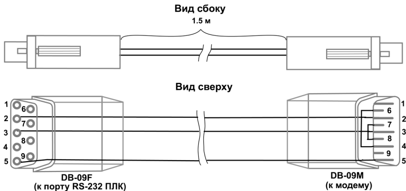
Рисунок Б.6 – Схема кабеля подключения модема к ОВЕН ПЛК100 по интерфейсу RS-232
