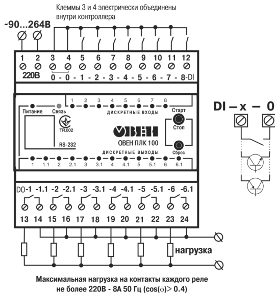
Рисунок Б.3 – Схема подключения питания, дискретных входов и выходов к ОВЕН ПЛК100-220.Р
